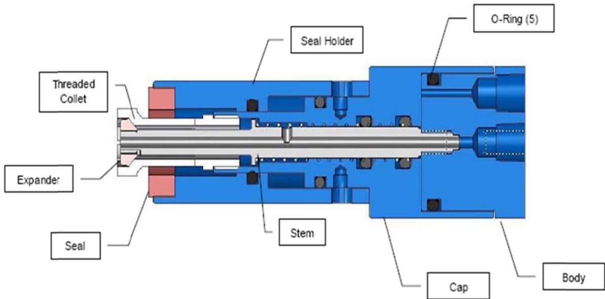
커넥터 조립 상세도
